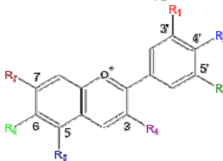
Antocianidinek
