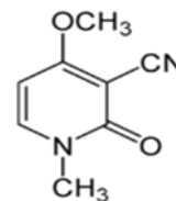
A ricinin szerkezete
